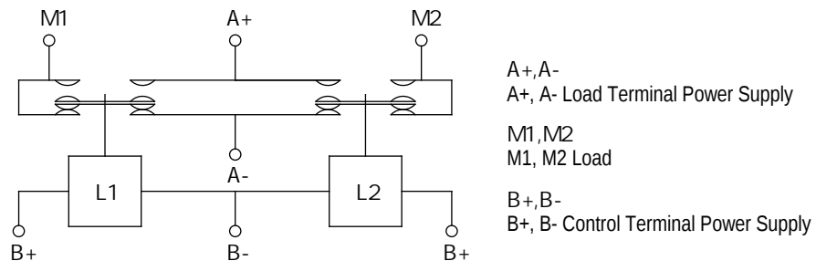
ADC50D ADC50D Wiring Diagram
